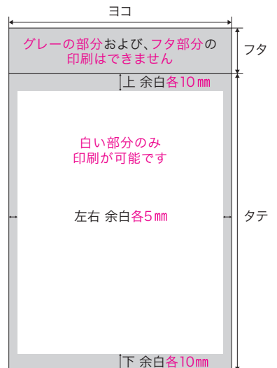
オフセット印刷 余白と印刷可能部分
