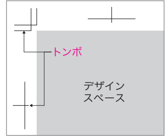
グラビア印刷 余白と印刷可能部分
